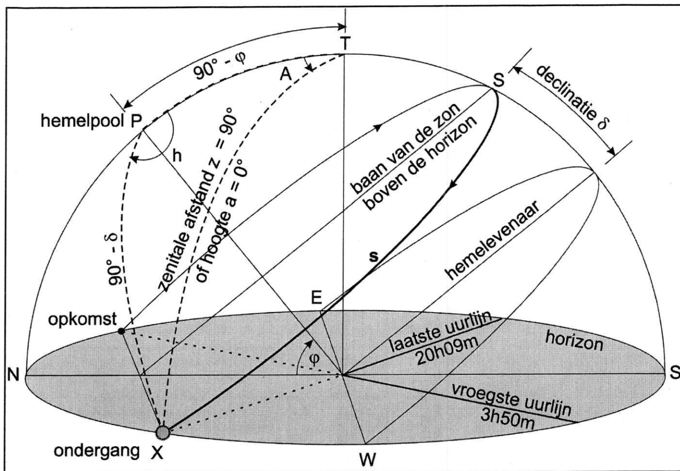
Figuur 1: baan van de zon boven de horizon op 21 juni voor een waarnemer op 51^\circ\text{N} .
